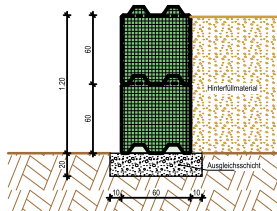
Pos. 1.4.2 - Betonstein 80
