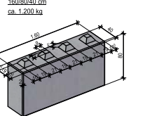
Betonbaustein
