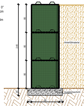
Pos. 1.4.3 - Betonstein 80
