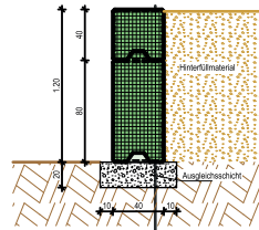
Pos. 1.3.2 - Betonstein 60
