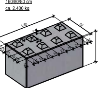
Betonbaustein
